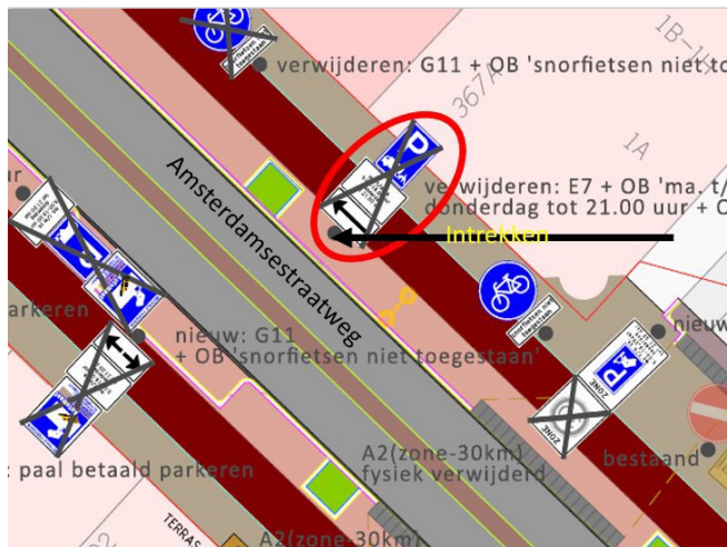
Uitsnede bebordingsplan
