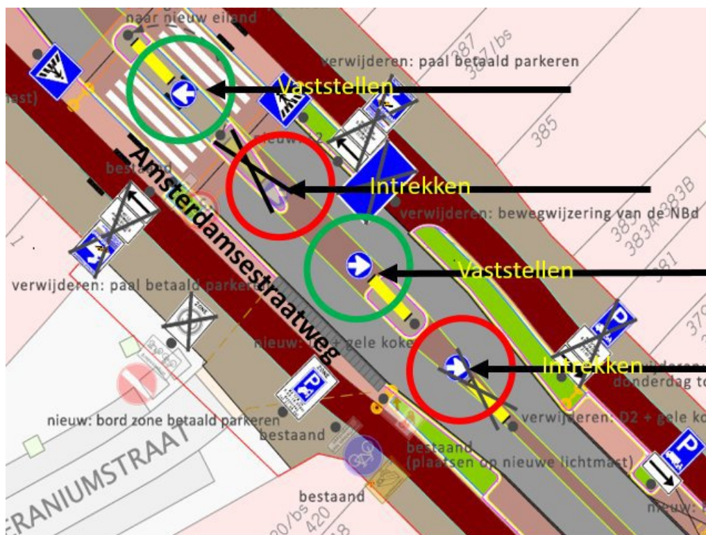
Uitsnede bebordingsplan
