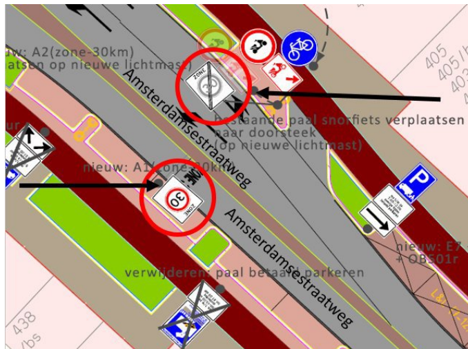
Uitsnede bebordingsplan
