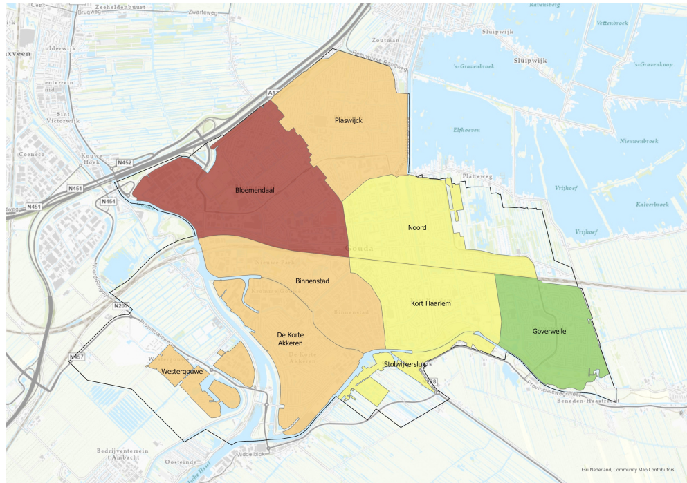
Afbeelding 5.15: Luchtkwaliteit (stikstof)
