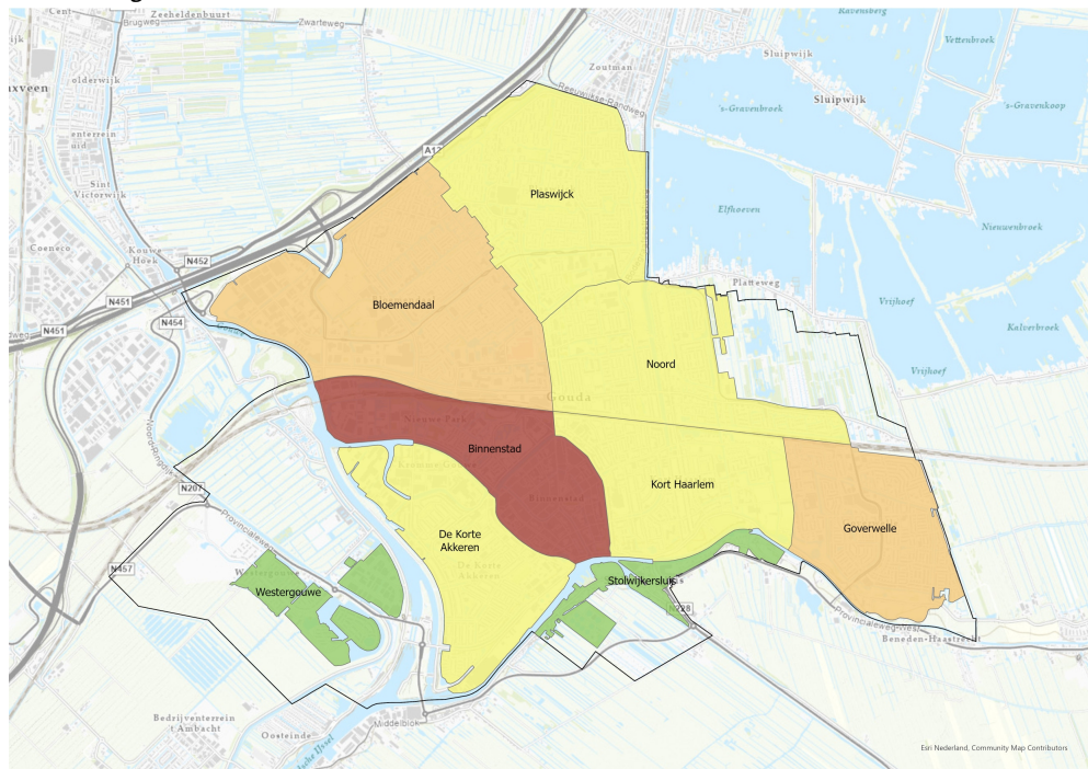
Afbeelding 5.15: Luchtkwaliteit (stikstof)
