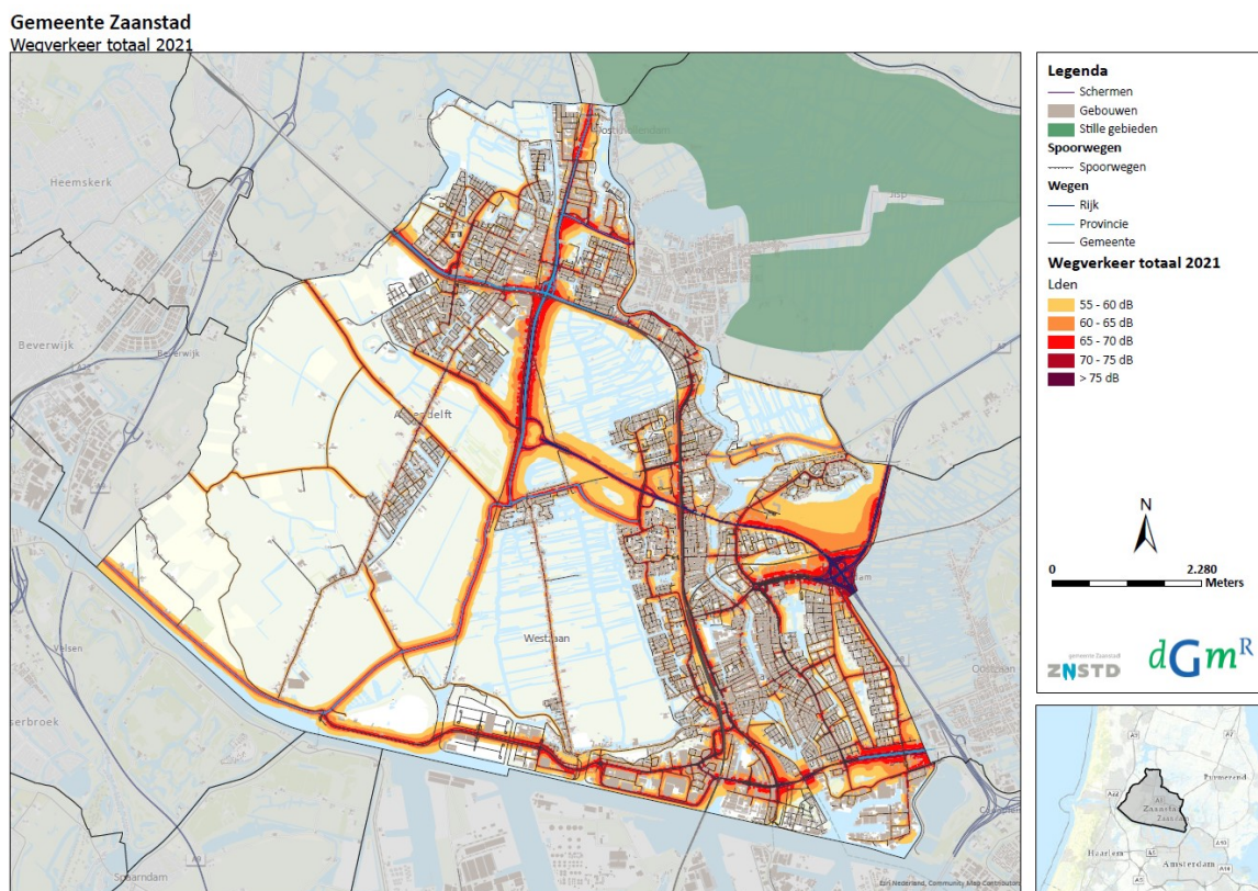
Geluidbelastingkaart Wegverkeer totaal 2021
