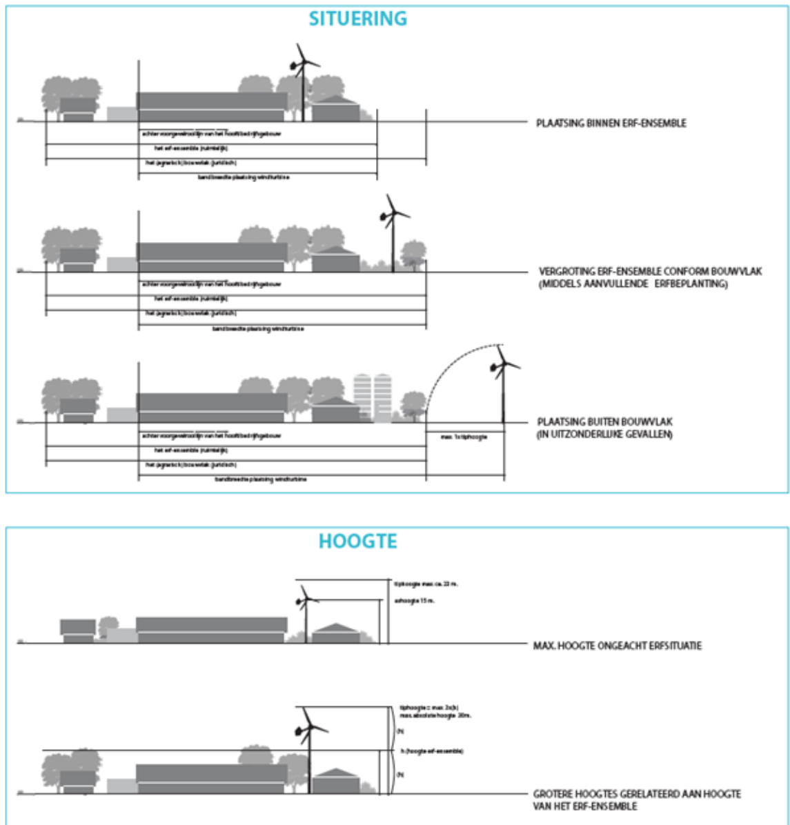
Afbeelding 2: Visualisatie inpassing windmolen t.o.v. het erfensemble
