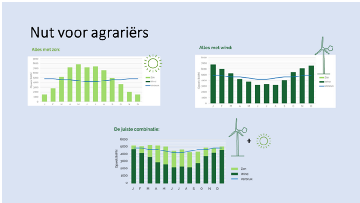
Afbeelding 6: Gunstige effect combinatie wind- en zonenergie (Bron EAZ)
