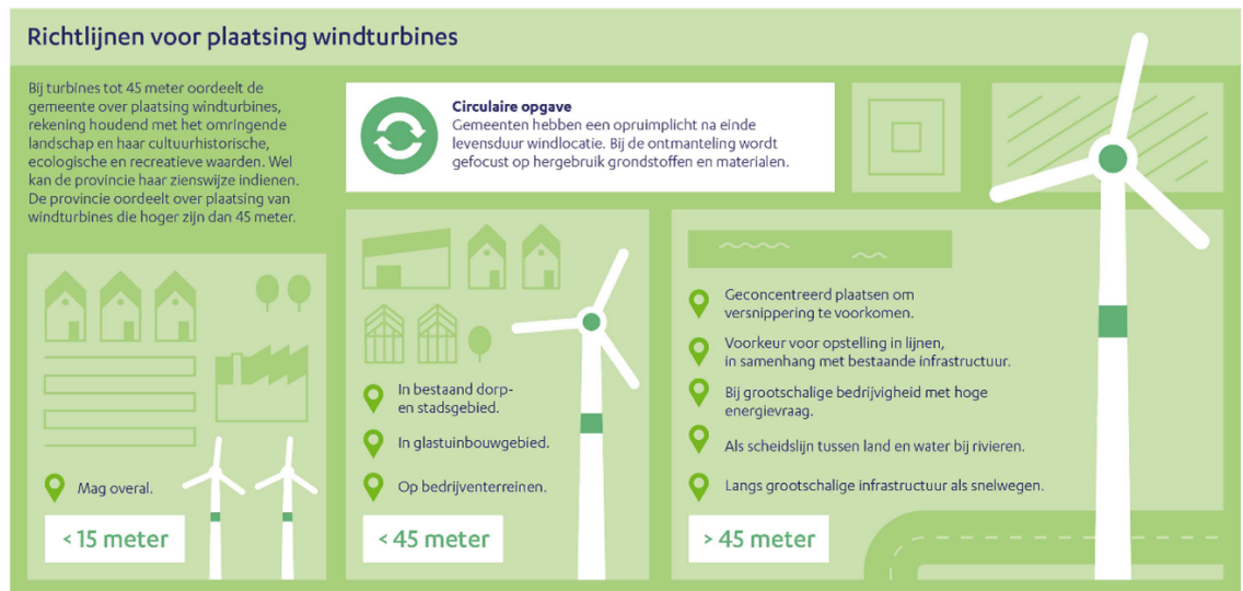
Afbeelding 1: Richtlijnen voor plaatsing windturbines (Bron: Provincie Zuid-Holland)
