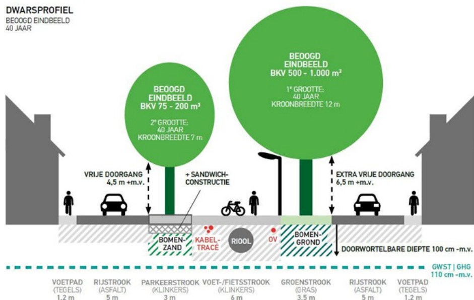
Dwarsprofiel straat met bomen. Bron: Norminstituut Bomen.
