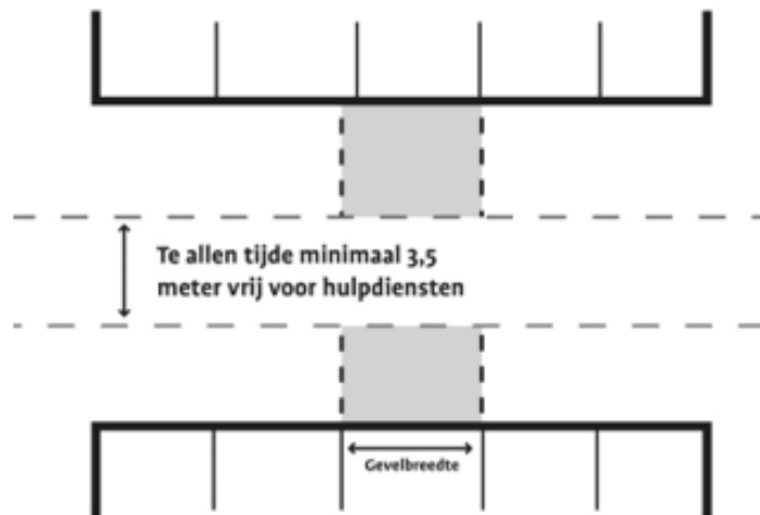
Figuur 3: principetekening gevelterras; ruimte vrijhouden voor hulpdiensten.
