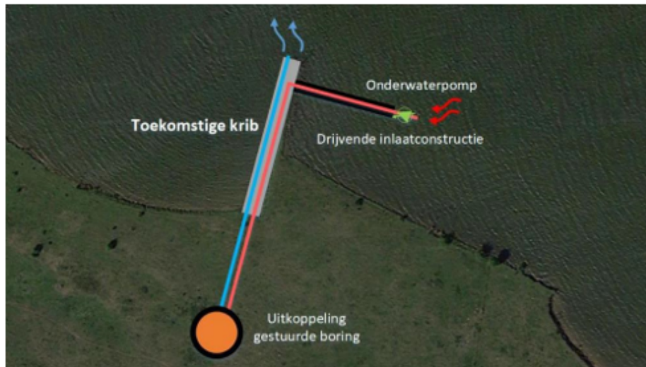
Figuur 4.3. Schetsontwerp aquathermie installatie (inlaat en uitlaat)
