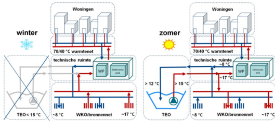
Figuur 4.1. Beoogd warmteconcept
