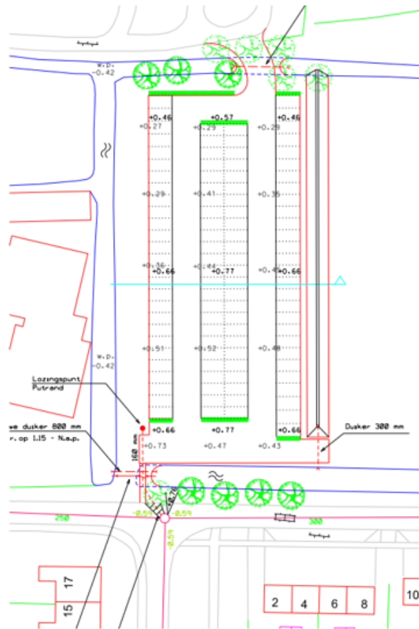
Aansluitpunt vuilwater
