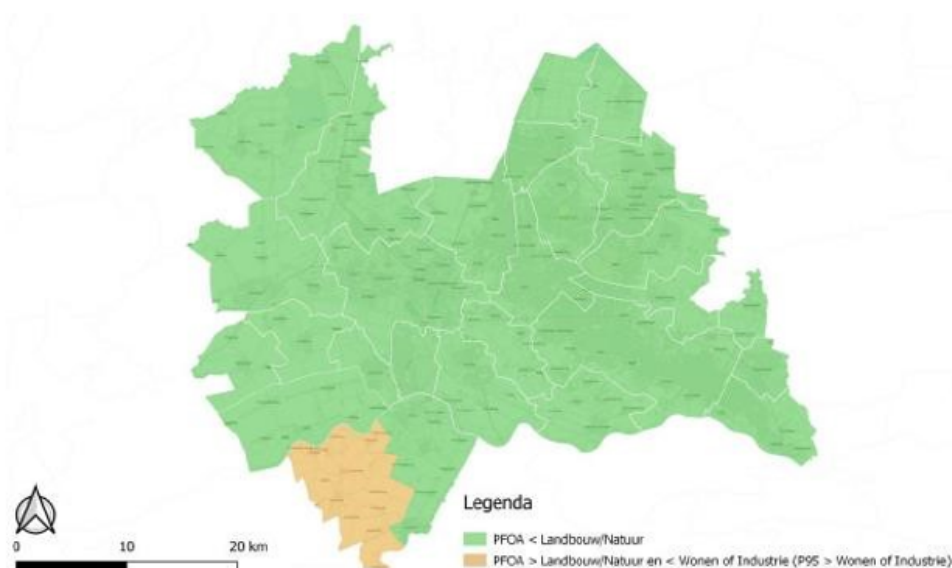
Figuur 3: PFOA ondergrond (0,5 – 2,0 m-mv)
