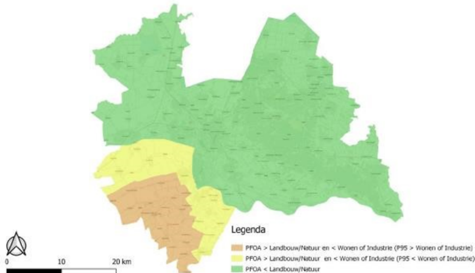
Figuur 2: PFOA bovengrond (0,0 – 0,5 m-mv)
