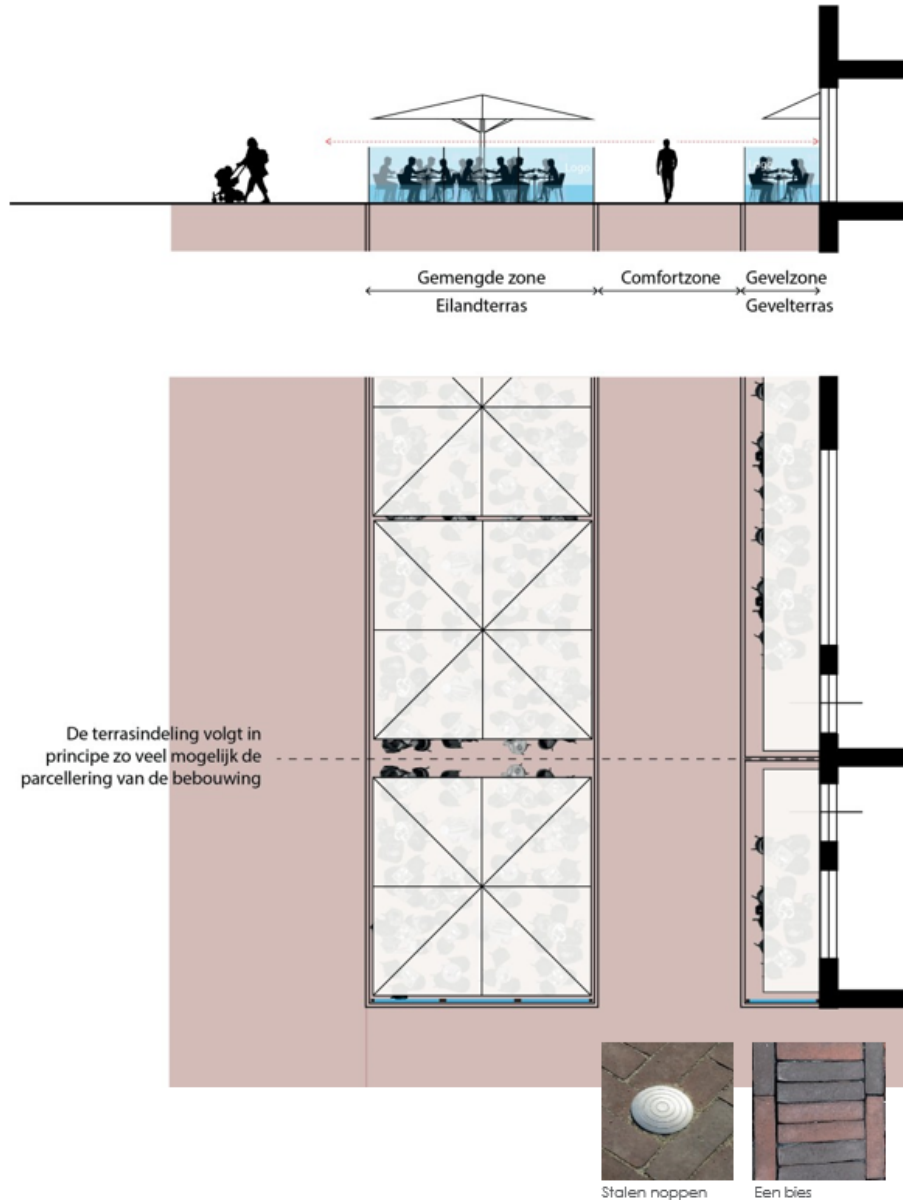
Afbeelding 3: Principedoorsnede opbouw terras
