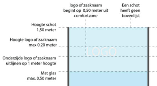
Afbeelding 9: Verschijningsvorm schot
