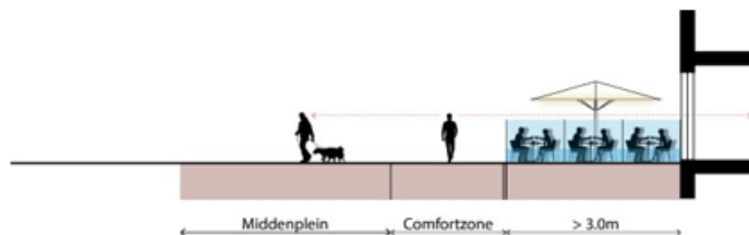
Afbeelding 7: Principedoorssnede opstelling parasol gevelterras > 3 meter
