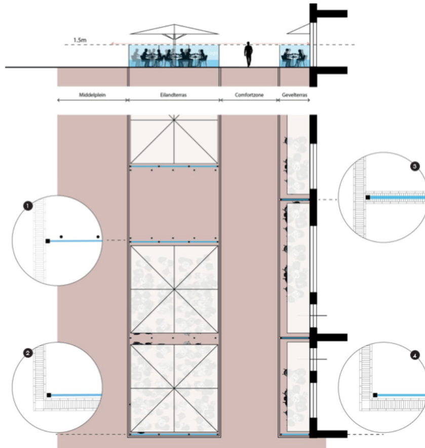
Afbeelding 10: Principeopstelling schotten in eilandterras en gevelterras
