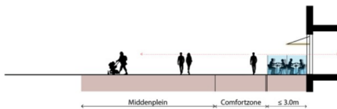
Afbeelding 6: Principedoorssnede opstelling luifels gevelterras 3 meter
