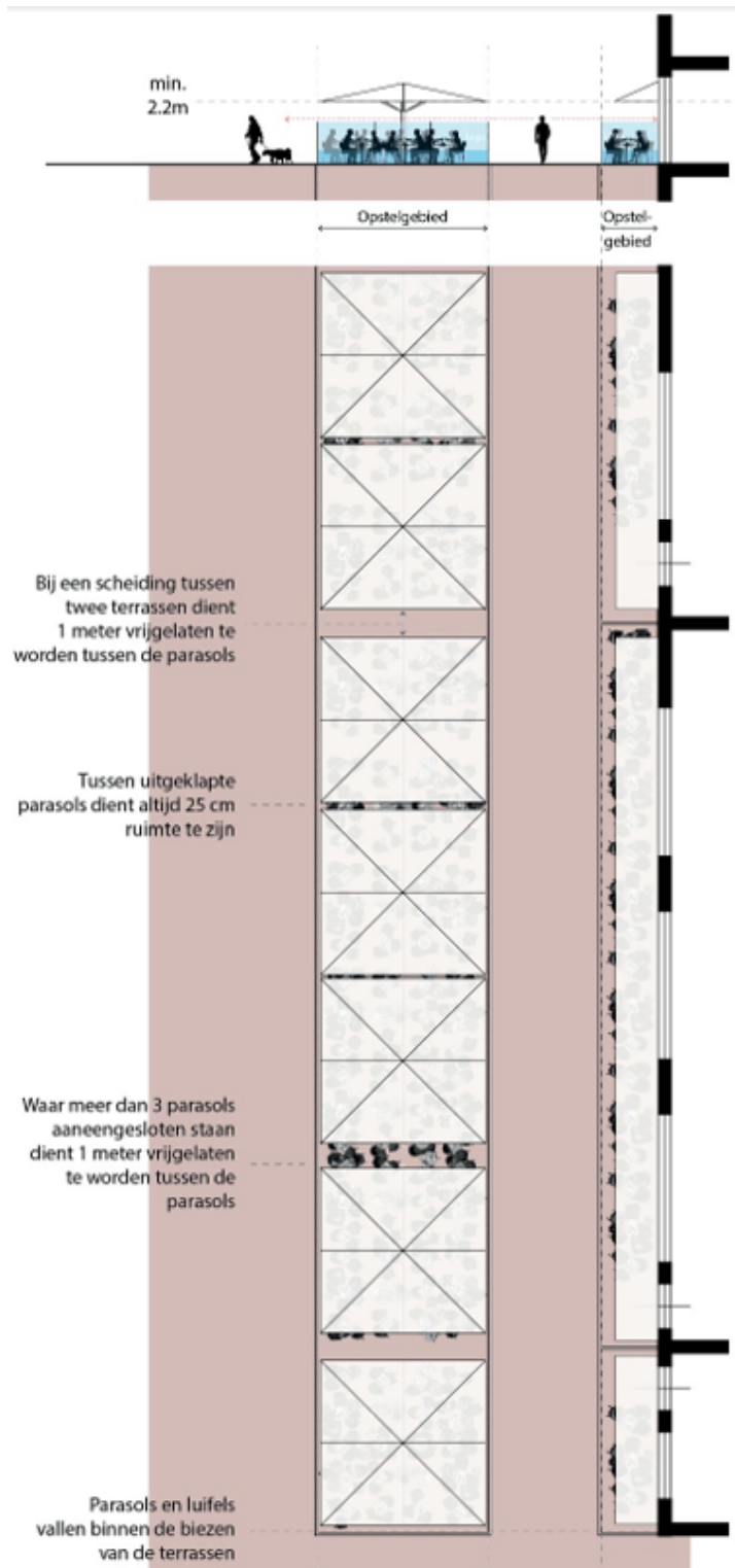
Afbeelding 8: Principedoorsnede opstelling parasol
