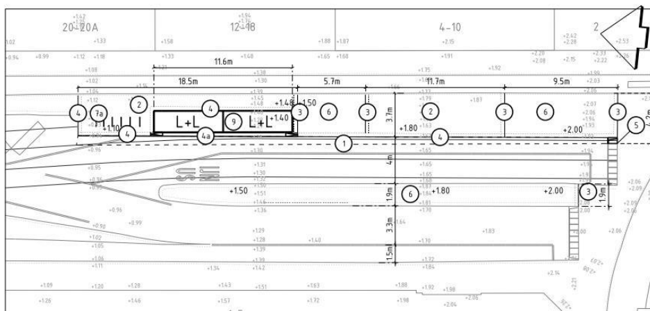
Nieuwe Situatie SCHAAL 1 : 200
