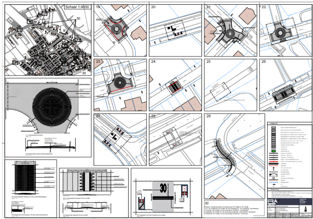
- GVVP-03-TEK-02 (blad 2), 30 zone Rossum, verhardingstekening blad 2
