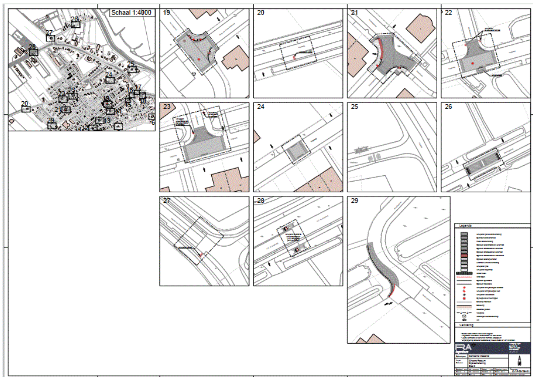
- GVVP-03-TEK-02 (blad 1), 30 zone Rossum, verhardingstekening blad 1
