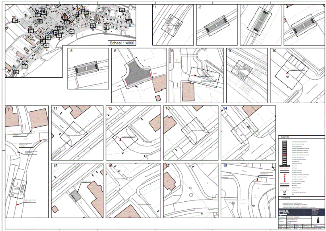
- GVVP-03-TEK-01 (blad 2), 30 zone Rossum, opbreektekening blad 2
