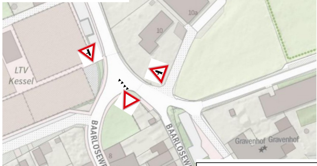
Toekomstige voorrangsregeling Kruispunt Baarloseweg – Markt - Ondersteweg
