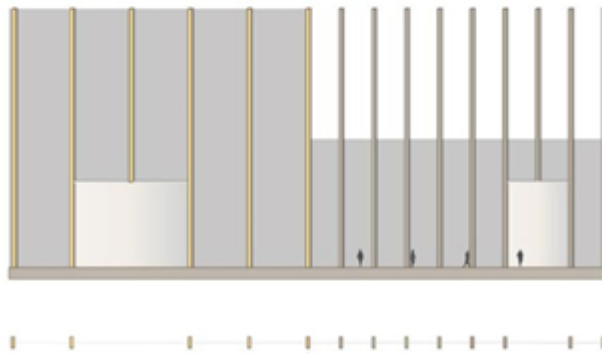
Verandering in de stramienmaat en andere kleurtint/materiaal
