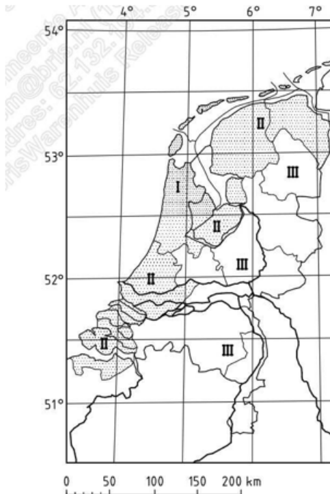
Figuur NB.1 — Indeling van Nederland in windgebieden
