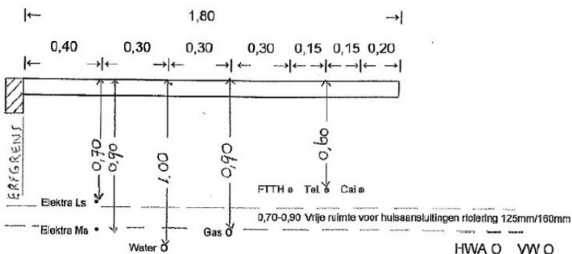
2. Normaal profiel trottoirs
