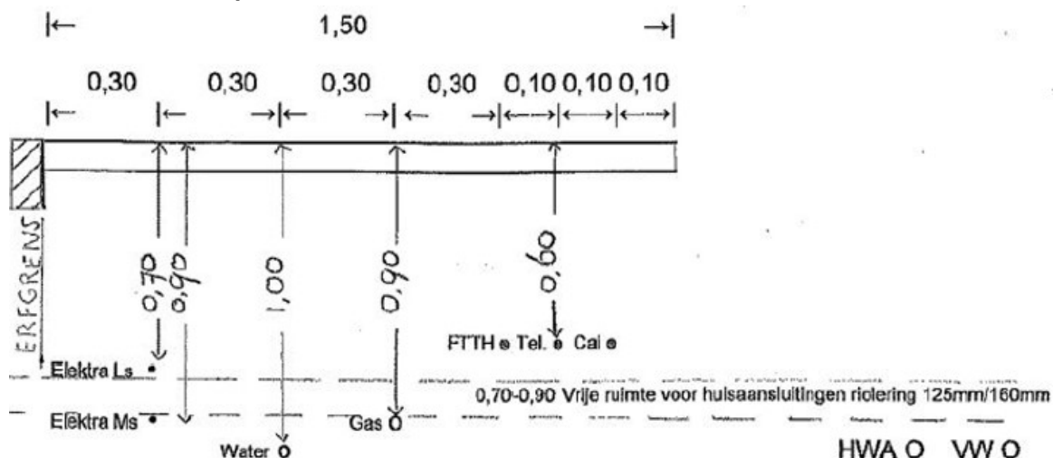
1. Normaal (small) profiel trottoirs
