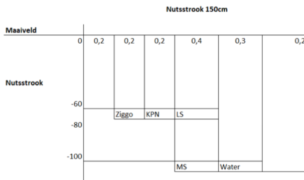
Afbeelding 2: Normprofiel exclusief gas
