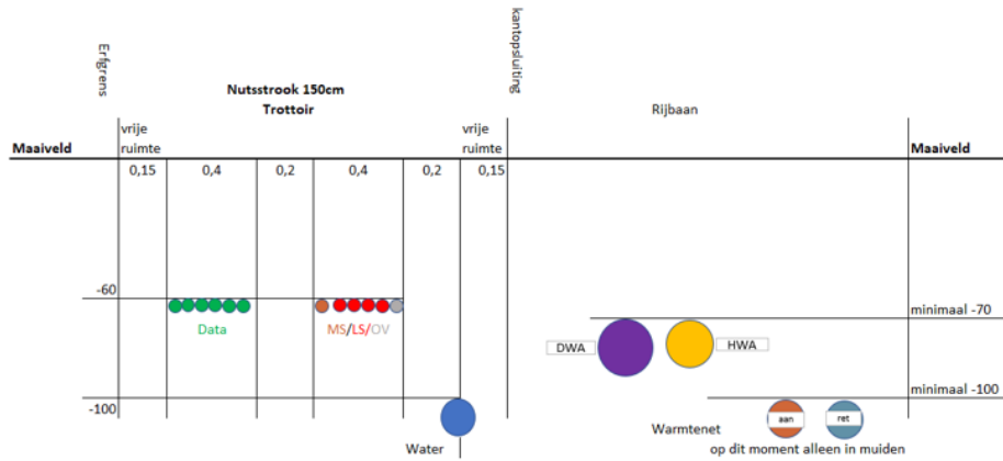
Afbeelding 1: Normprofiel inclusief gas
