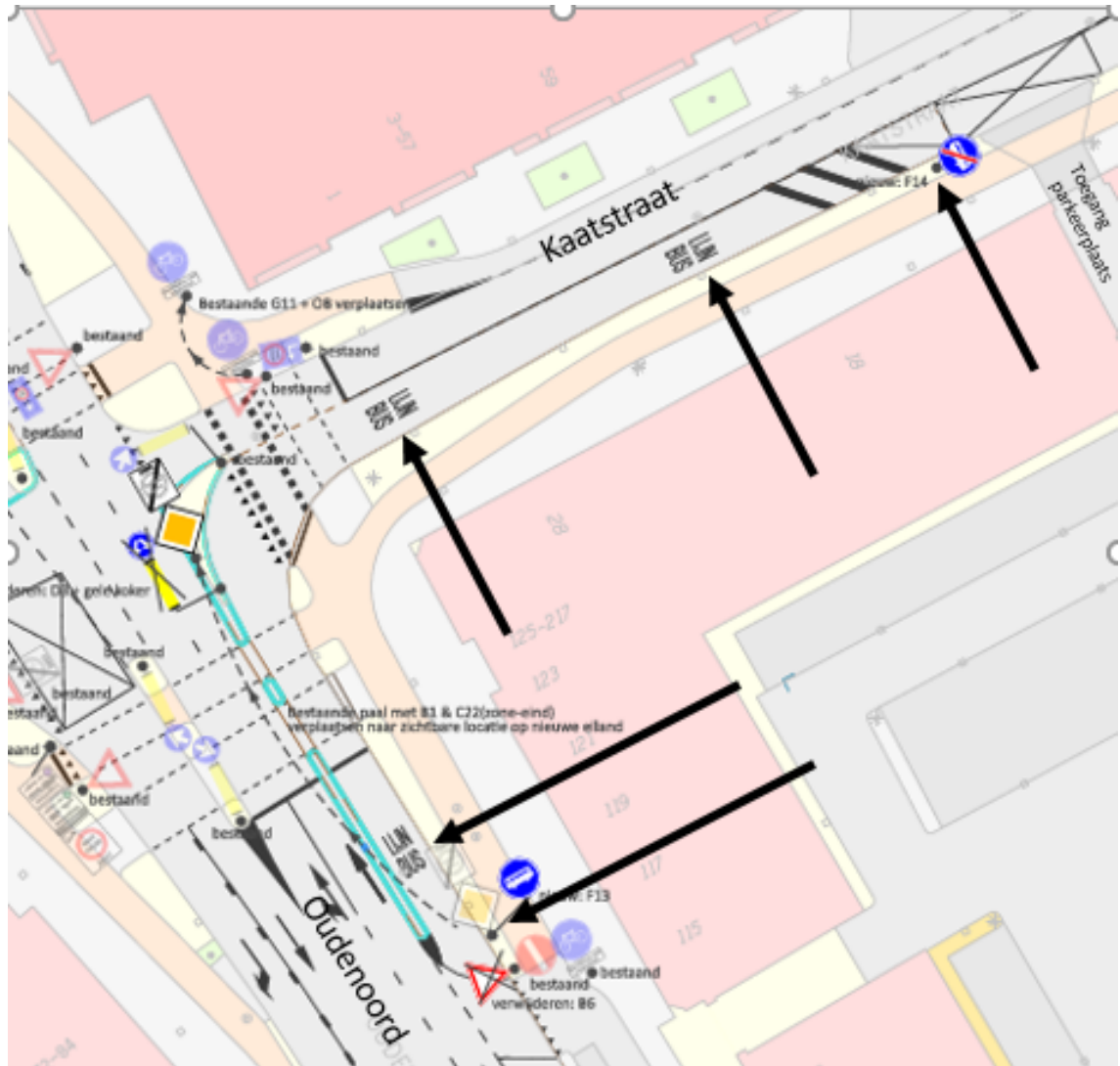
Uitsnede bebordingsplan
