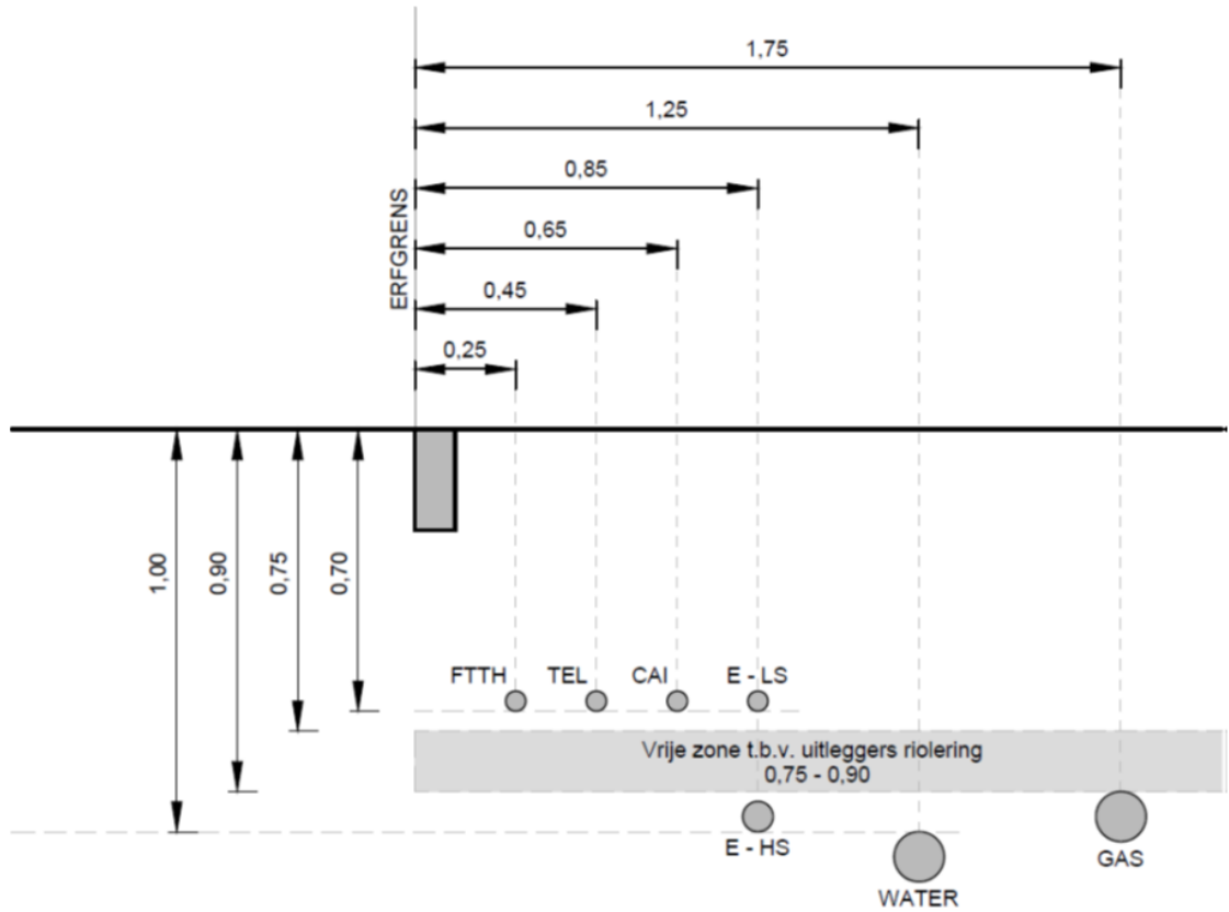
Figuur 1 - Standaard dwarsprofiel 01 (FTTH en telecom)
