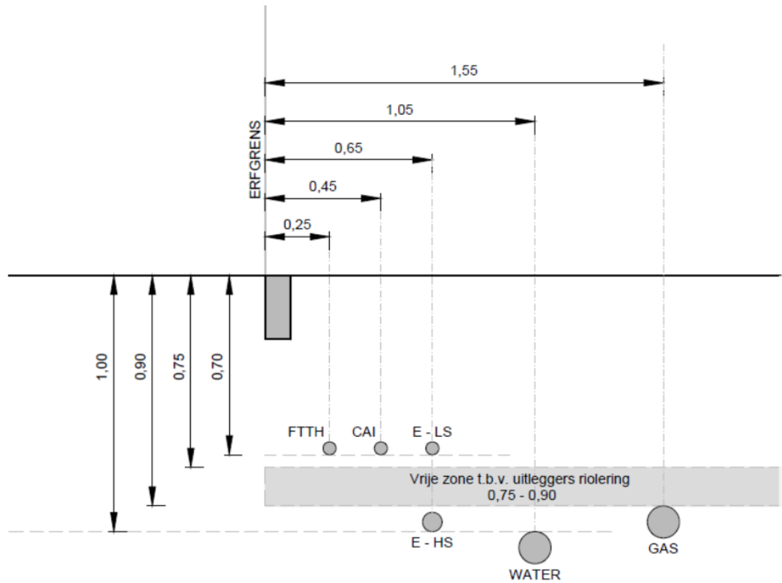
Figuur 2 - Standaard dwarsprofiel 02 (alleen FTTH)
