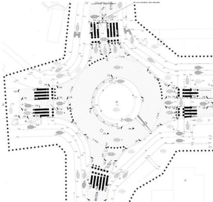
Situatietekening ZD22035700-2. Aanleggen voetgangersoversteekplaatsen bij rotonde Antwerpseweg – Kon. Julianastraat te Rijsbergen, door plaatsing van borden L2 van bijlage I van het Reglement verkeersregels en verkeerstekens 1990 met de daarbij behorende markering.
