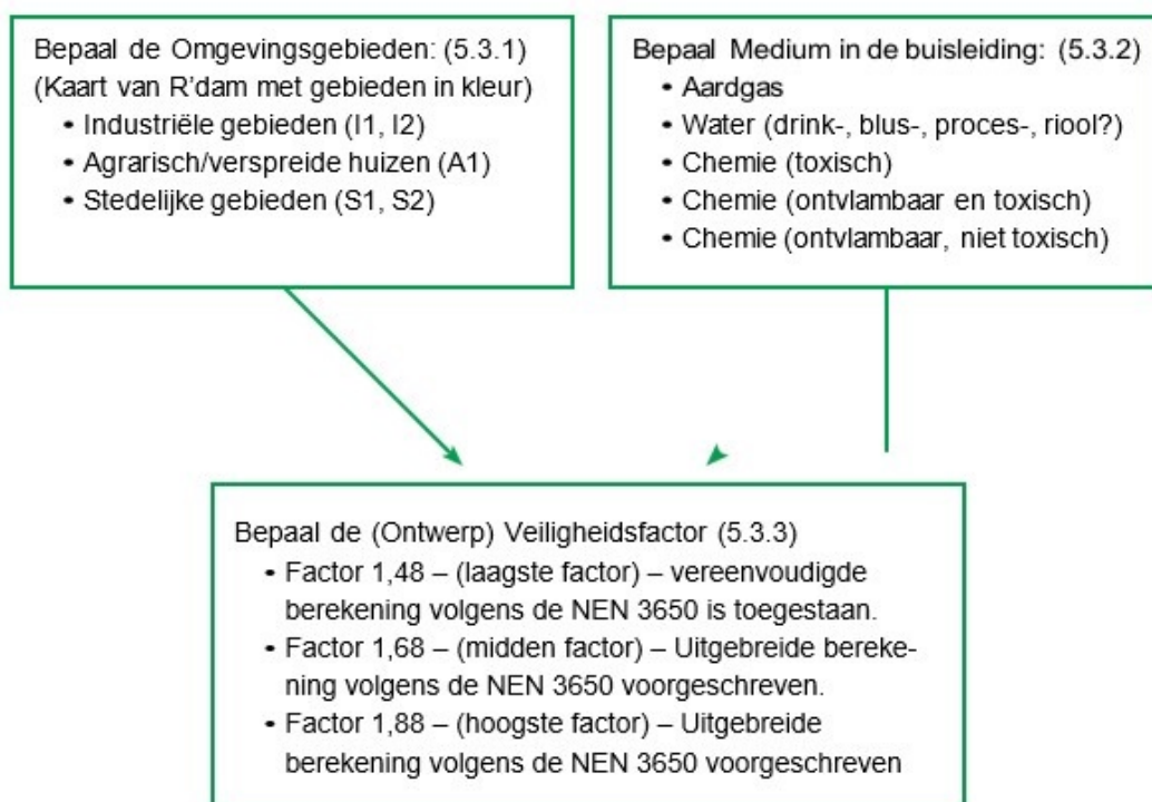
Figuur 4, Bepaling van de (Ontwerp) Veiligheidsfactor
