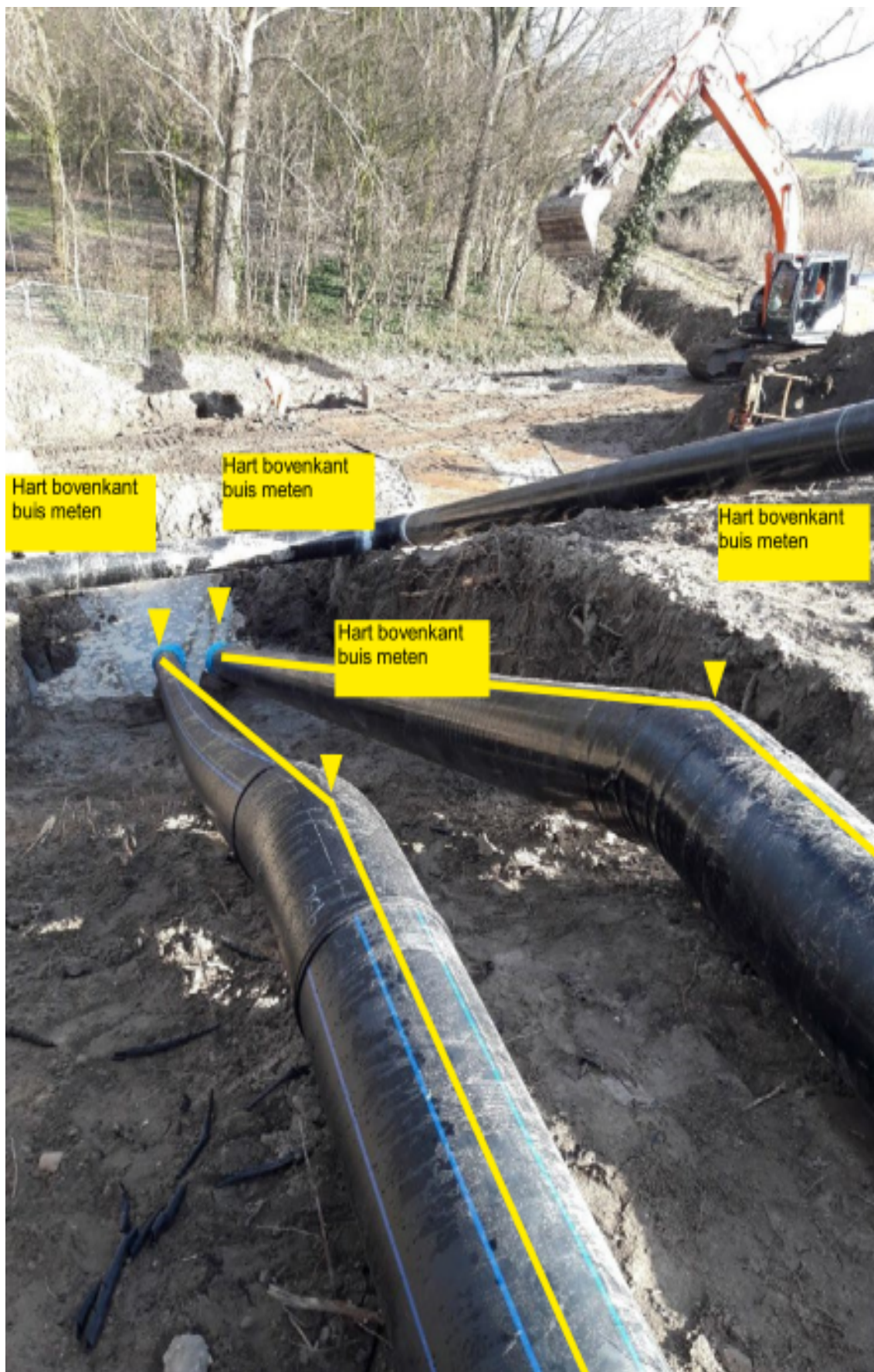
Voorbeeld van benodigde tussenpunten in verband met verandering in hoogte.
