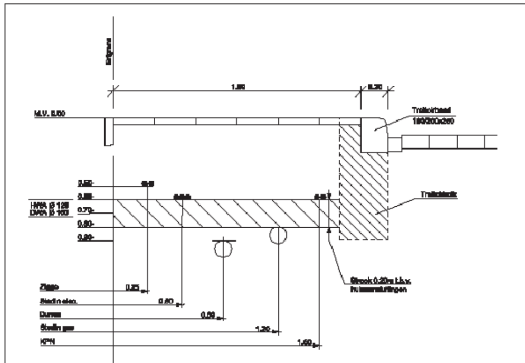
Standaardprofiel kabels en leidingen oudere wijken bestaande situatie, trottoir 1.80 m breed schaal 1 : 20
