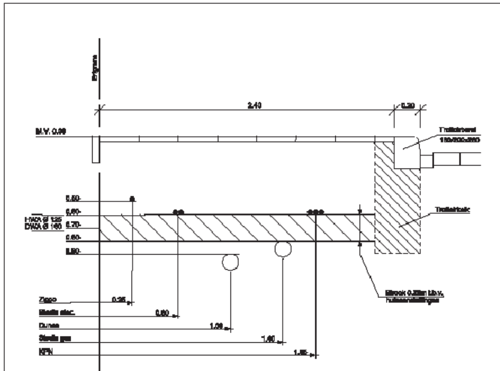
Standardprofiel kabels en leidingen oudere wijken bestaande situatie, trottoir 2.40 m breed
