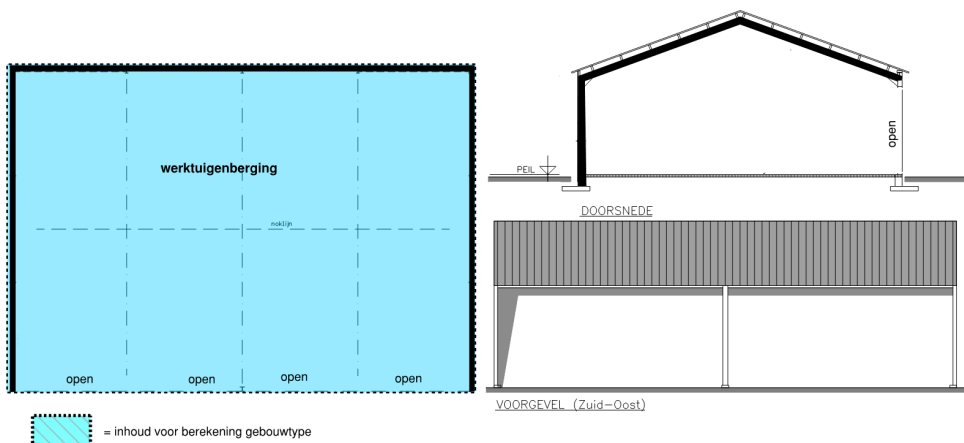
Oppervlakte gedeeltelijk open werktuigenloods
