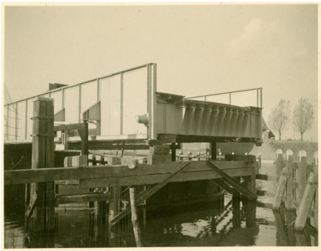
Afbeelding 3 Collectie: Groninger Archieven Beschrijving: Korrewegbrug; brugdek geopende toestand, Gerret Krolbrug Datum: 1954 Identificatienummer: NL-GnGRA_2544_3565
