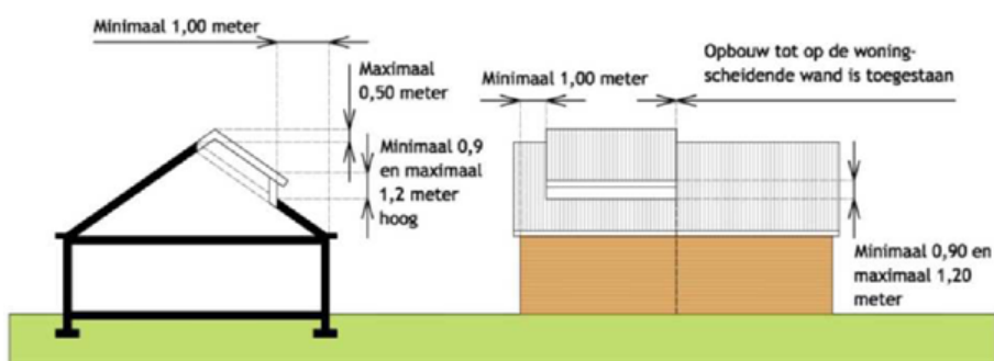
Voorbeeldsituatie artikel 6.2.1 in combinatie met artikel 6.2.4
