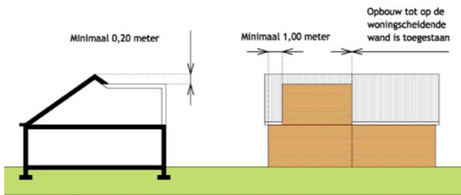
Voorbeeldsituatie artikel 6.2.1 in combinatie met artikel 6.2.4
