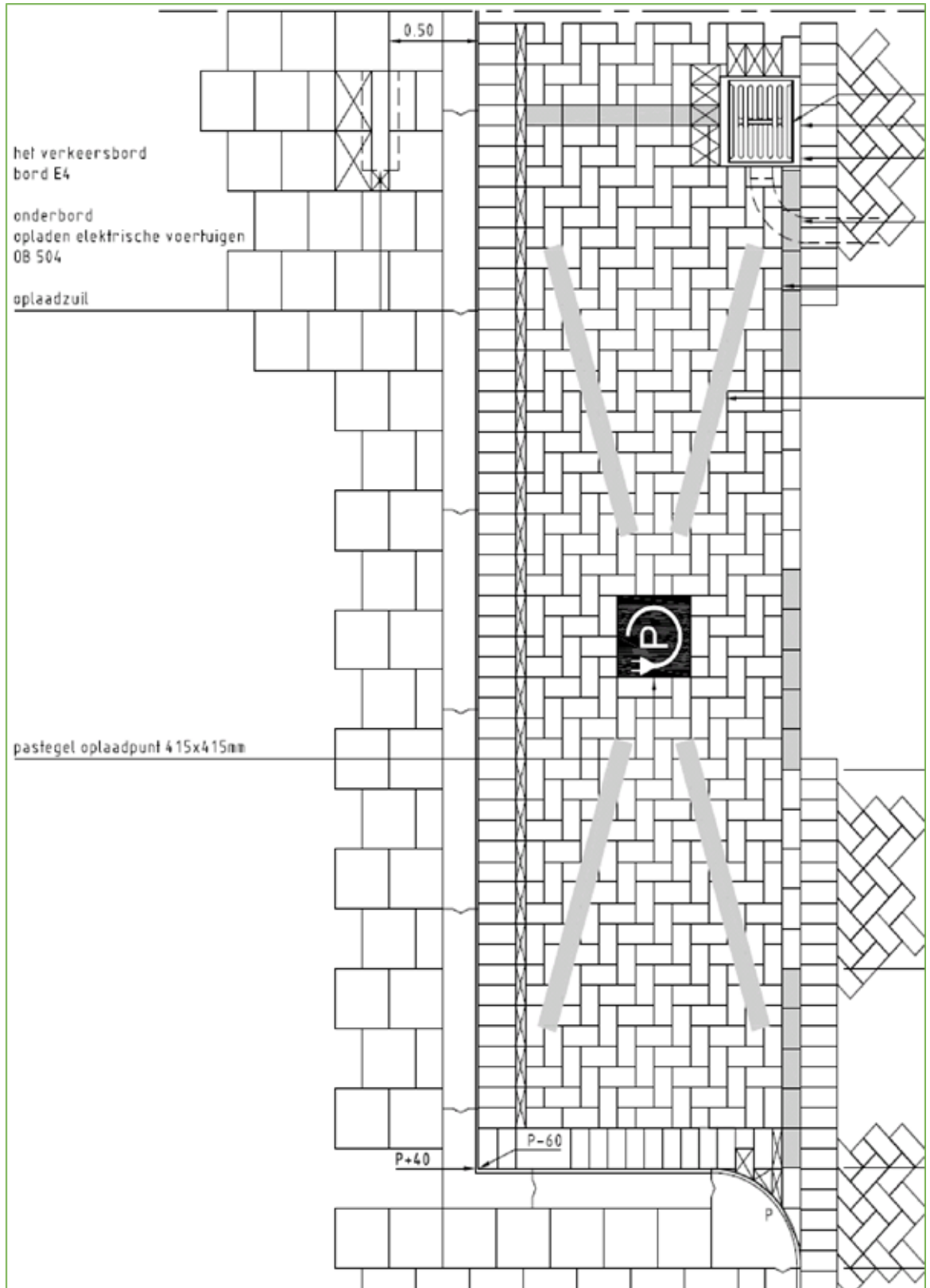
Figuur 3: Inrichting laadvakken bij langsparkeren
