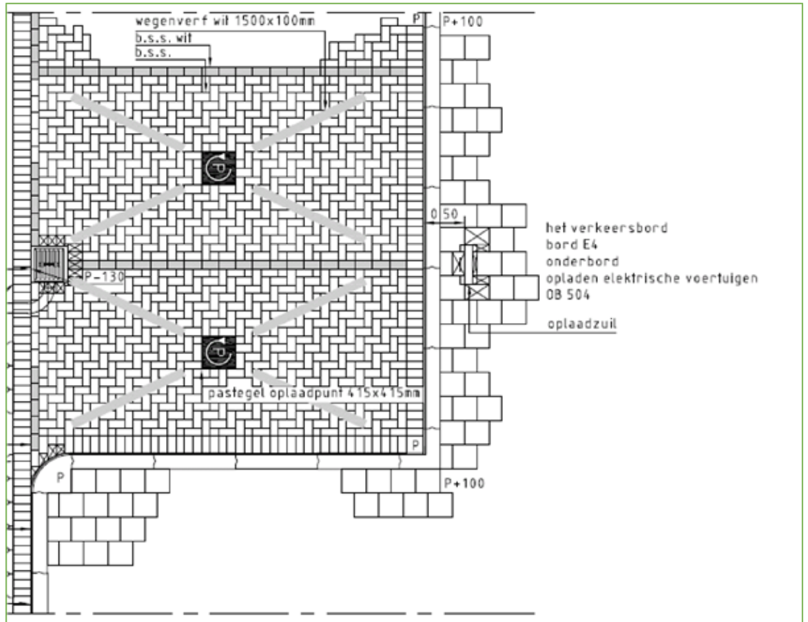
Figuur 4: Inrichting laadvakken bij haakparkeren
