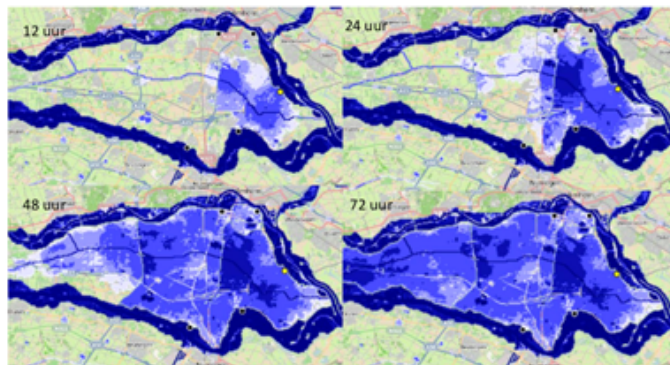
Figuur 3-2 Inundatieverloop bij Toetspeil scenario (Tp) Angeren na 12, 24, 48 en 72 uur na doorbraak van de waterkering nabij Angeren aan de oostzijde van het gebied (voorbeeld van een van de vijf doorbraakscenario's).
