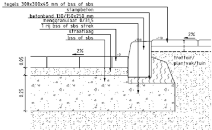
(A) Trottoirband langs bestrating of parkeerplaats
