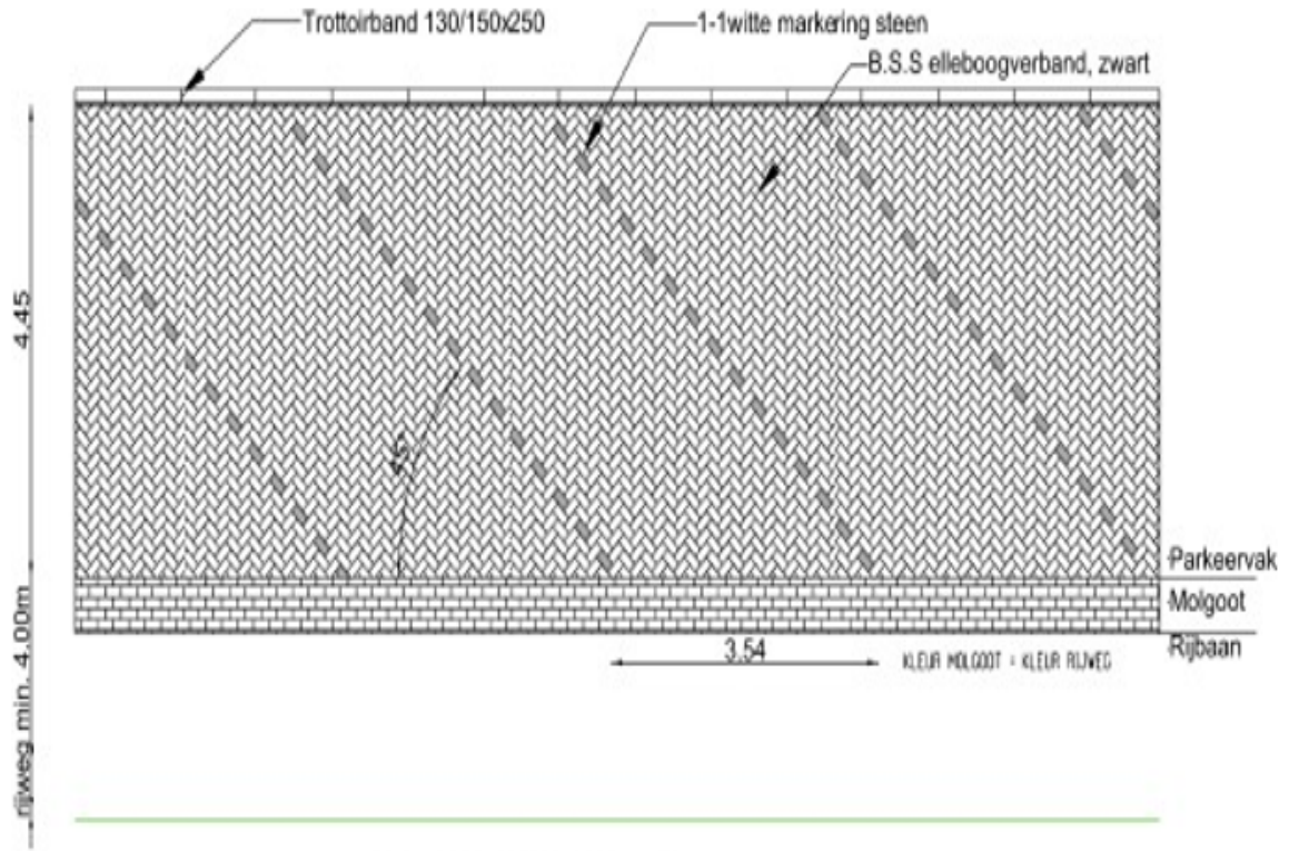
DETAIL SCHUINPARKEREN 45°
