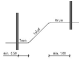
Dwarsdoorsnede Talud met OV-masten
