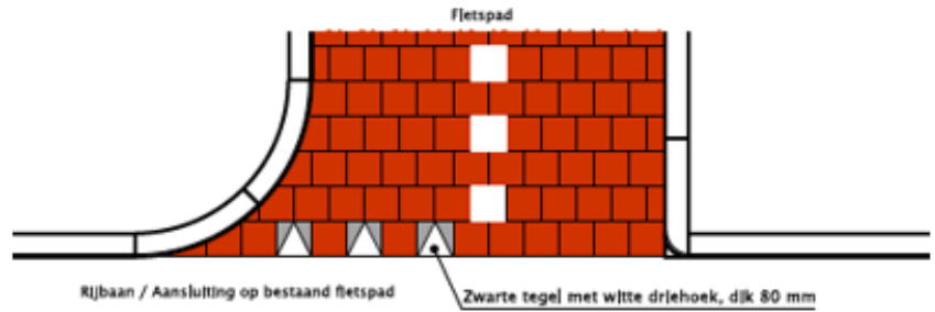
FIETSPAD
