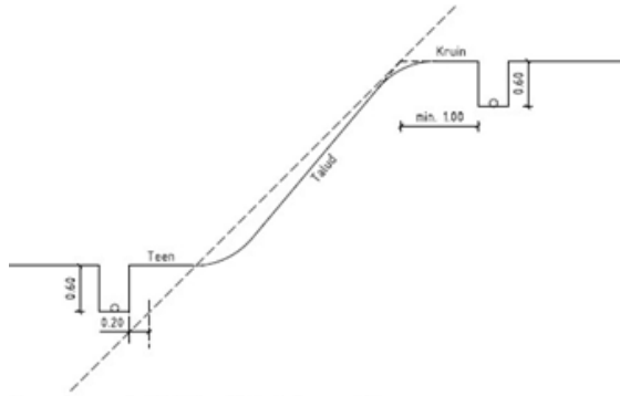
Dwarsdoorsnede Talud met kabelsleuven OV
