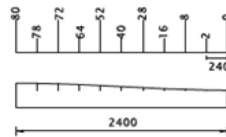
LENGTEPROFIEL
