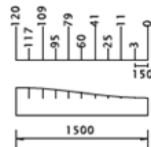
LENGTEPROFIEL
