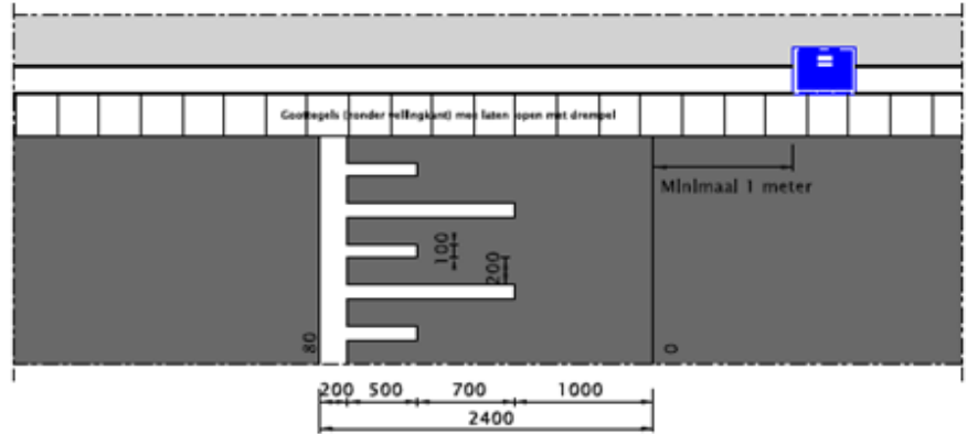
MARKERING ASFALTDREMPEL
