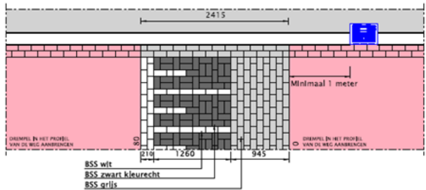
MARKERING ASFALTDREMPEL
