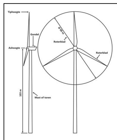
Figuur 2 uitleg begrippen windmolen
