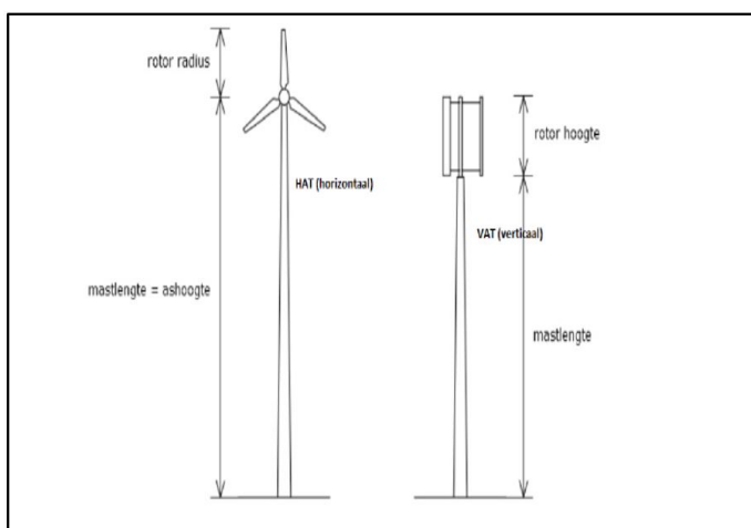
Figuur 1 soorten kleine windmolens
