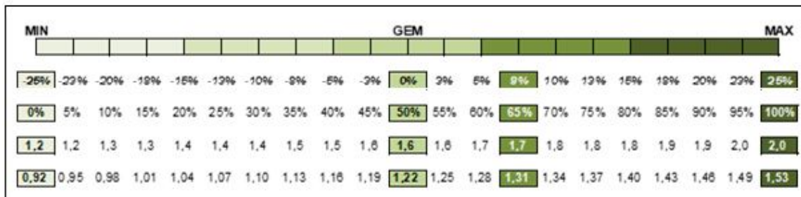
Figuur 1 Bepalen parkeernorm Barneveld t.o.v. bandbreedte CROW-kencijfers
