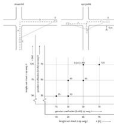
Figuur 10.1/11. Uitzichtdriehoeken
