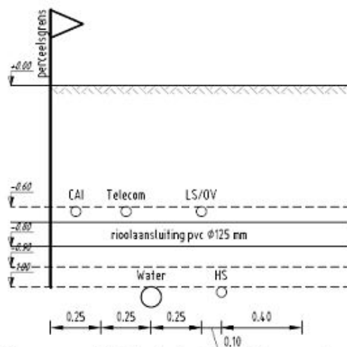
Dwarsprofiel kabels & leidingen nieuwbouw (gasloos)
