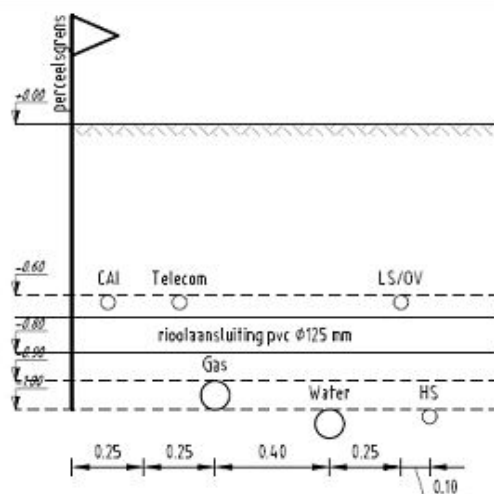
Dwarsprofiel kabels & leidingen inclusief gasleiding
