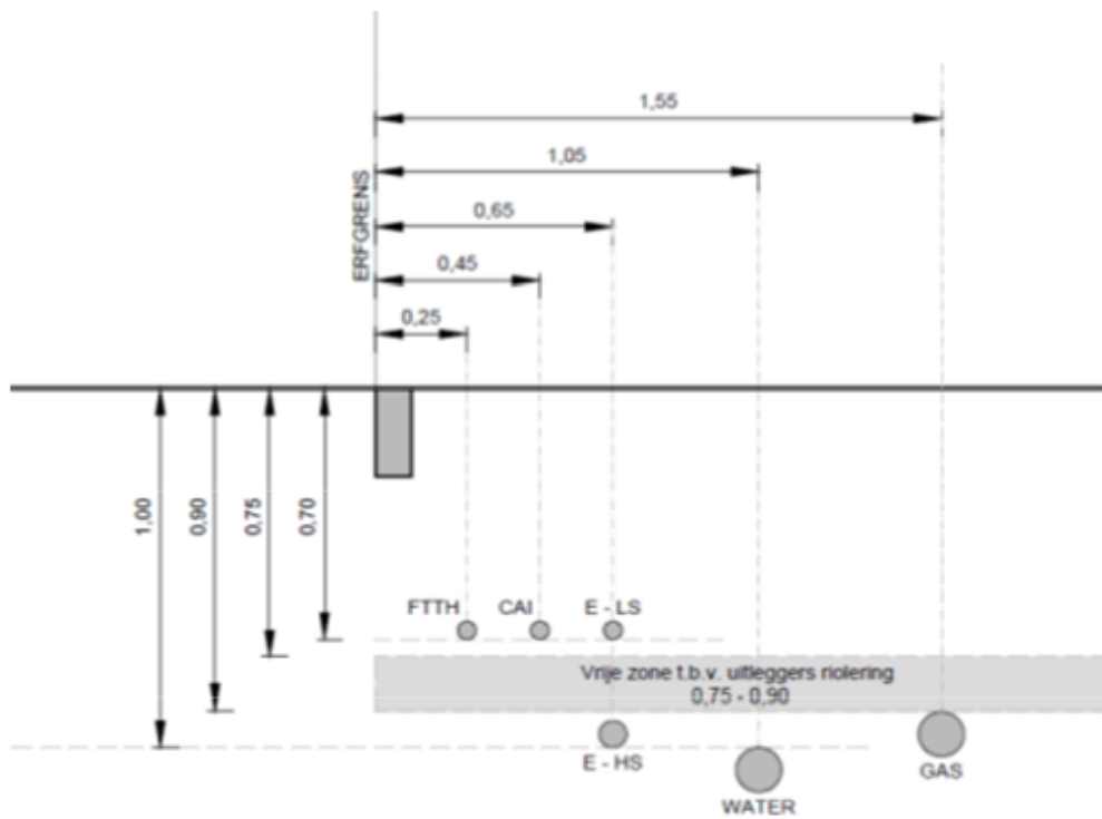
Figuur 2 - Standaard dwarsprofiel 02 (alleen FTTH)
