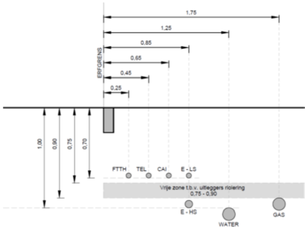
Figuur 1 - Standaard dwarsprofiel 01 (FTTH en telecom)
