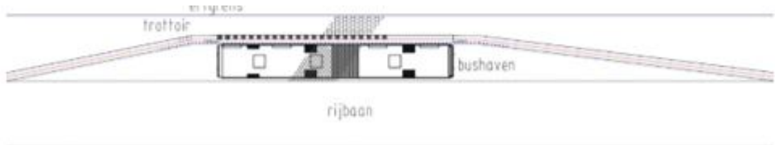
Figuur 2. Boven-aanzicht van een bushalte met haltekomp
