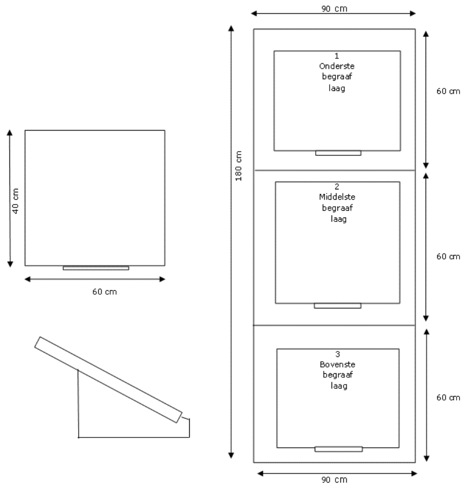
Figuur 4; gedenktekens op een algemeen graf in liggend vlak en zijaanzicht.
