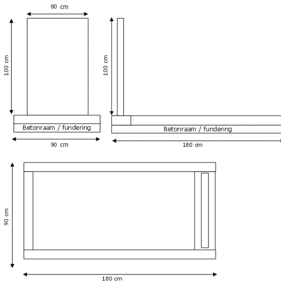
Figuur 1; Gedenkteken op een enkel particulier graf
