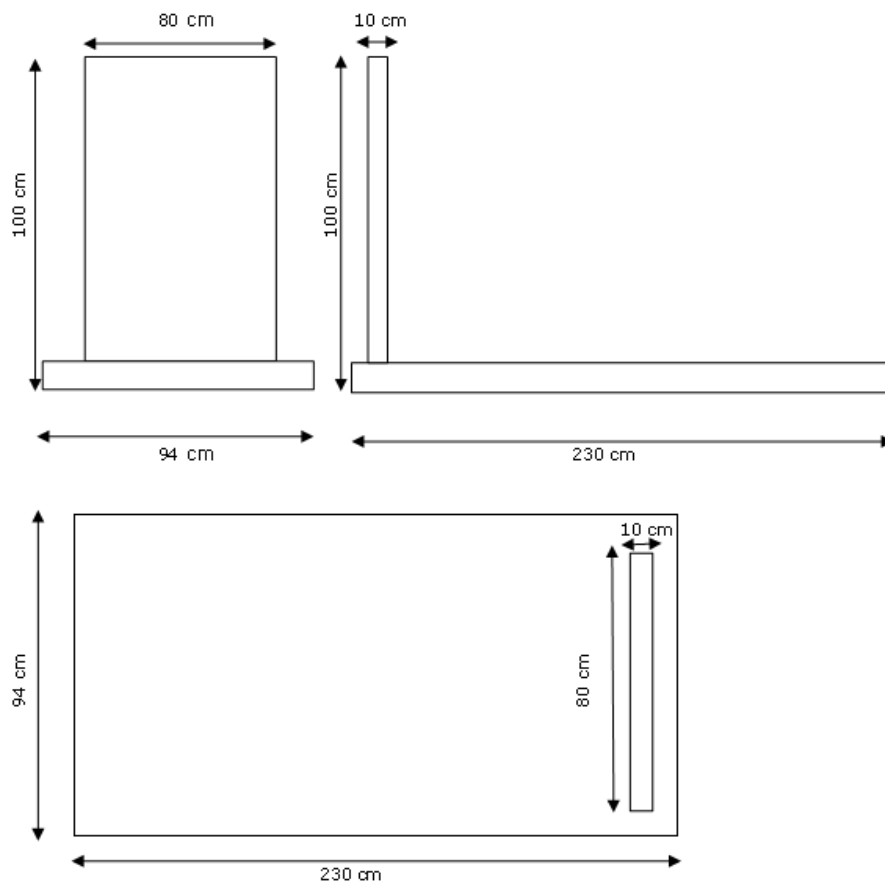
Figuur 2; Gedenkteken op een enkel keldergraf. Afmetingen in lengte en breedte kunnen iets afwijken van de praktijksituatie.
