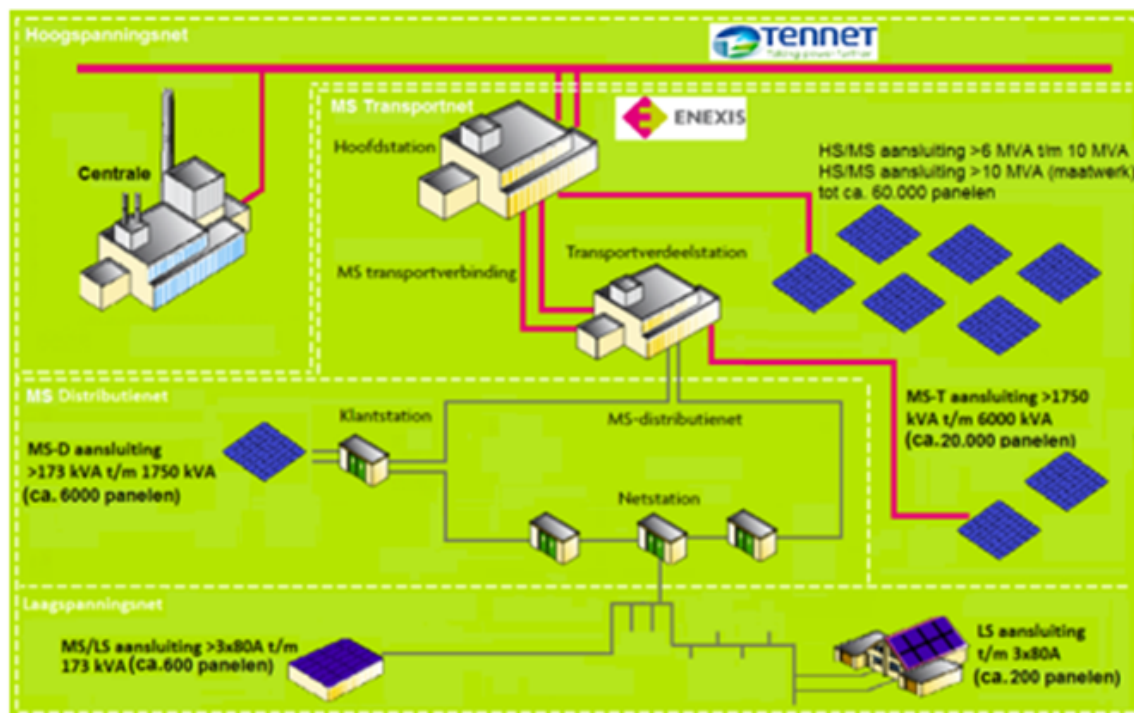
Figuur 5. Schematische weergave elektriciteitsnetwerk
