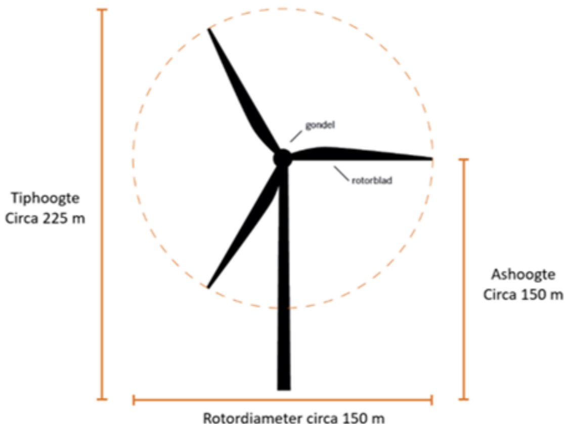
Figuur 2. Windturbine met definities
