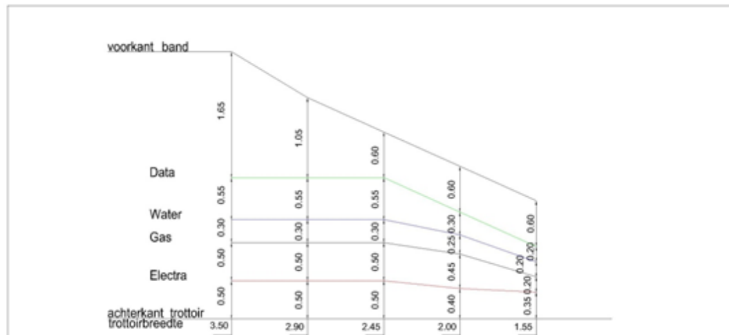
Bovenaanzicht schaal 1:50
