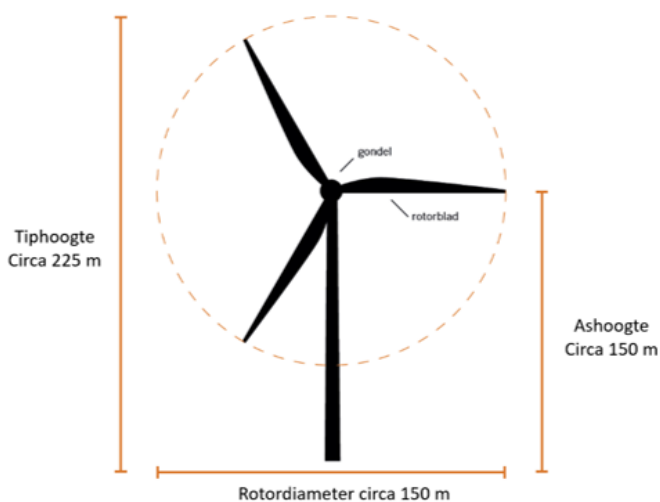
Figuur 2. Windturbine met definities
