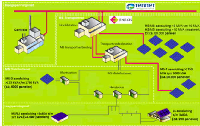
Figuur 5. Schematische weergave elektriciteitsnetwerk
