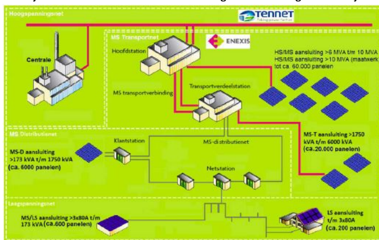
Figuur 5. Schematische weergave elektriciteitsnetwerk
