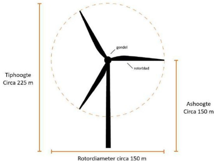
Figuur 2. Windturbine met definities
