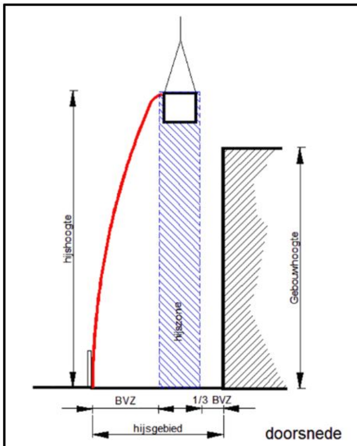
Figuur 4 – Extra bouwveiligheidsruimte
