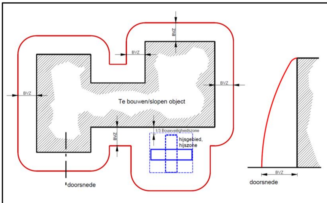
Figuur 2 - Bouwveiligheidszone met hijsg gebied
