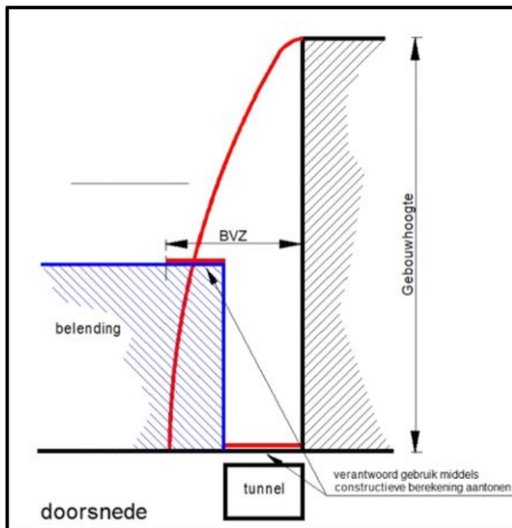
Figuur 6 – Doorsnede situering bouwveiligheidszone
