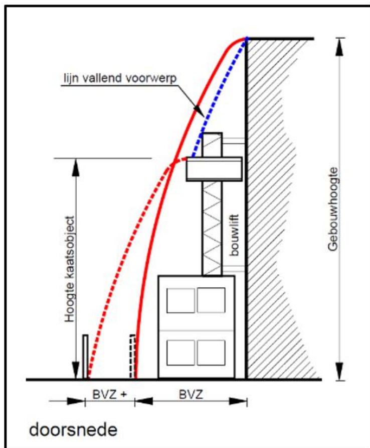
Figuur 7 – Uitbreiding bouwveiligheidszone bij afkaatsgevaar
