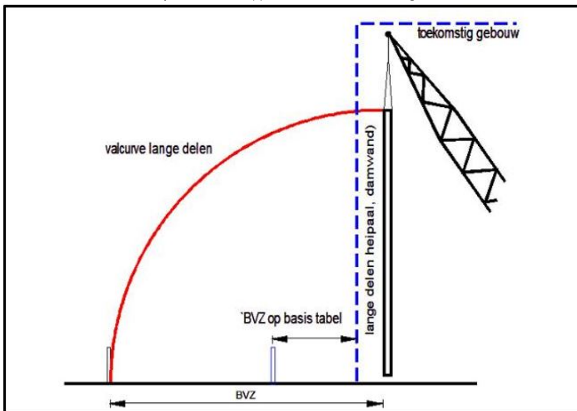
Figuur 8 – Bouwveiligheidszone bij lange delen
