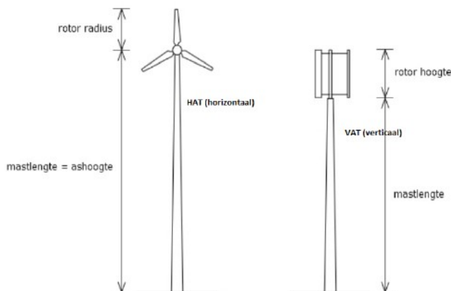
Figuur 1 – kleine windmolen, begrippen
