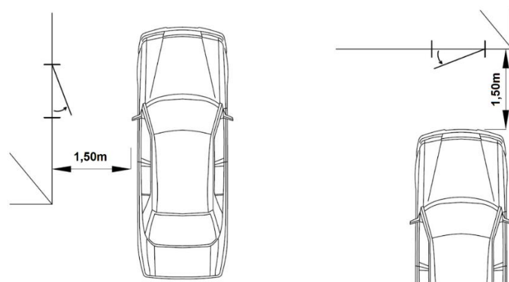
Figuur 14. Benodigde afstand tussen een parkeerplaats en een voordeur t.b.v. de loopruimte
