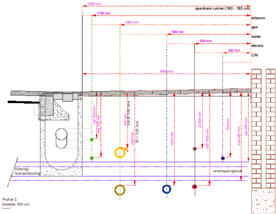
Profil 3, breedte 180 cm (woonerf)
