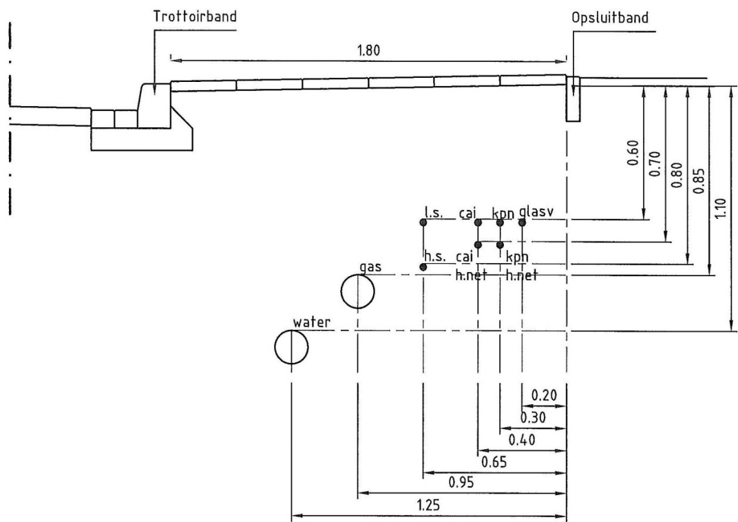
DWARSPROFIEL T.B.V. KABELS EN LEIDINGEN
