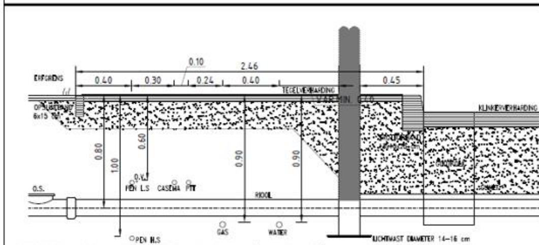
DWARSPROFIEL BIJ EEN TROTTOIRBreedTE VAN 2.46 m (MET LICHTMAST)
