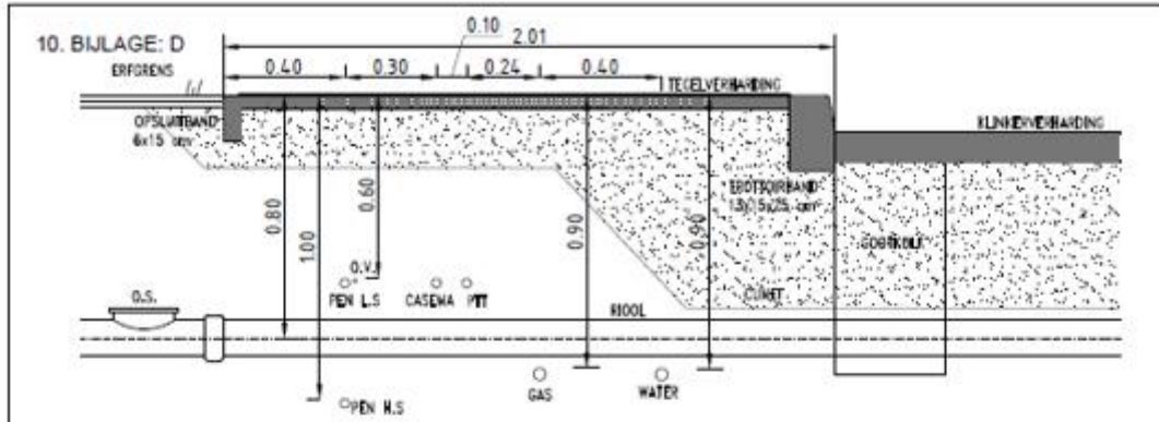
DWARSPROFIEL BIJ EEN TROTTOIRBreedTE VAN 2.01 m (ZONDER LICHTMAST)
