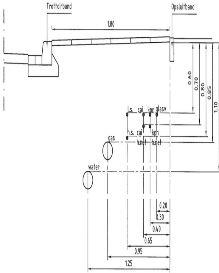
DWARSPROFIEL T.B.V. KABELS EN LEIDINGEN
