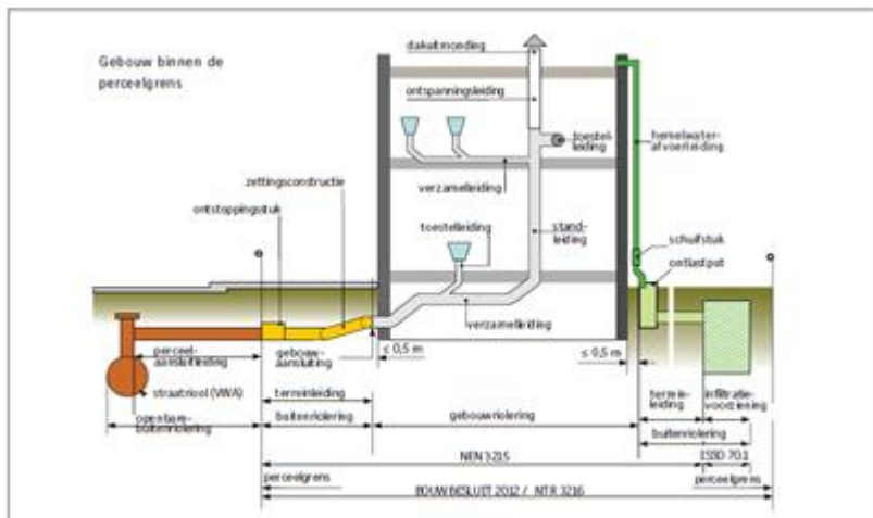
Figuur 1 Overzicht reikwijdte en definities bij woning met tuin en hemelwaterinfiltratie op eigen terrein
