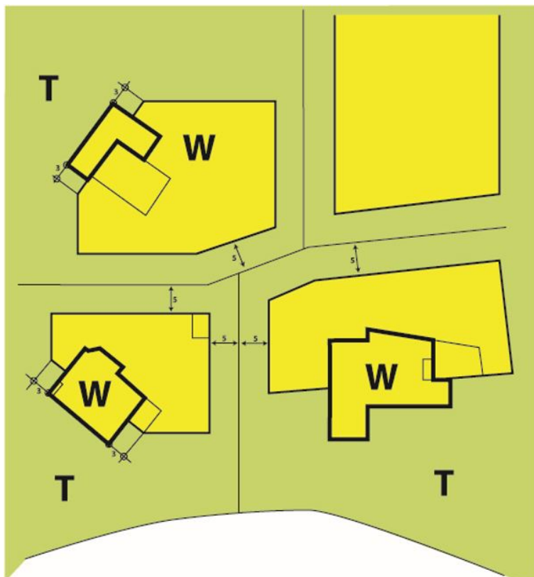
Figuur 10 Situatietekening gebiedstype 3
